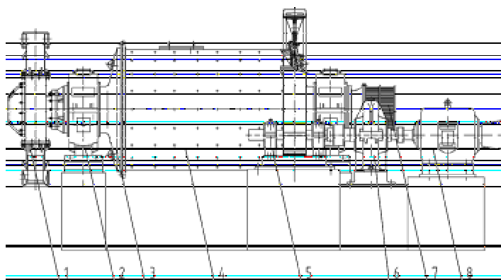
1. 联合给料部 2. 轴承部 3. 进料部 4. 筒体部 5. 传动部 6. 减速机 7. 出料部 8. 电动机
